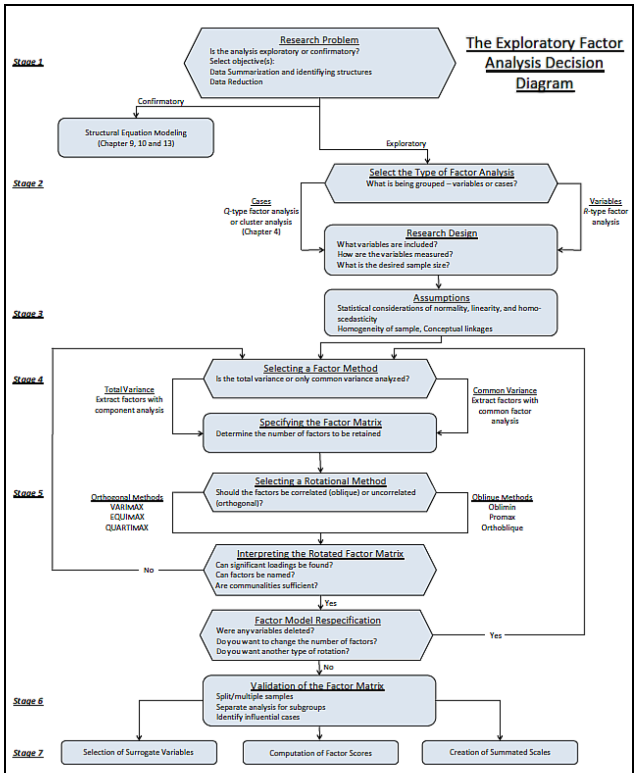
Slika 42. Dijagram toka eksplorativne faktorske analize. Izvor: Sarstedt, 2019., prema Hair i dr., 2014.
