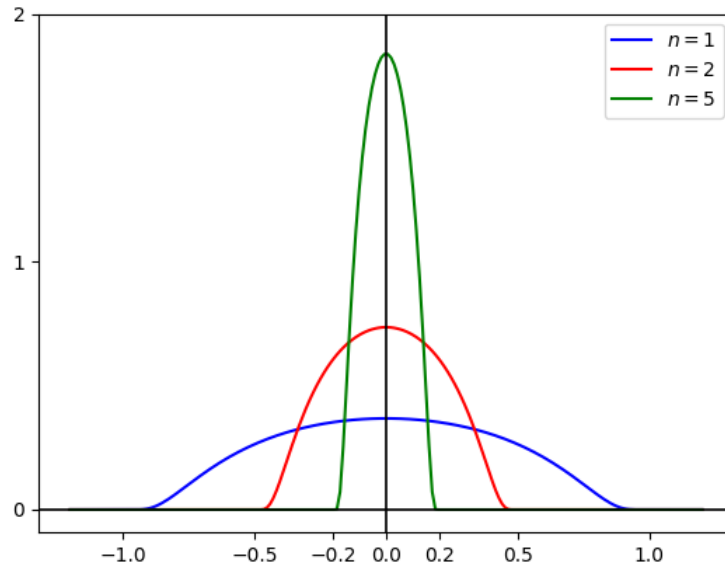
Slika 1: Grafovi funkcija \rho_1 , \rho_2 i \rho_5
