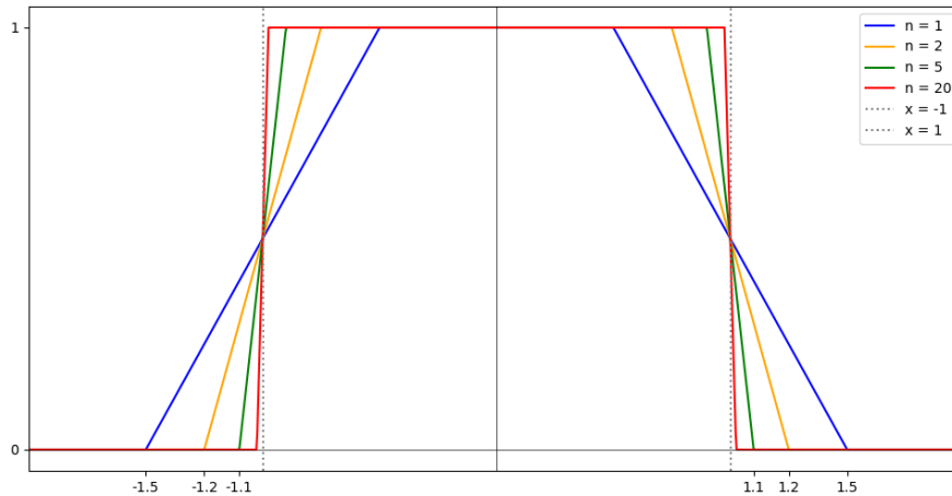
Slika 2: Graf funkcije f_n za nekoliko vrijednosti n
