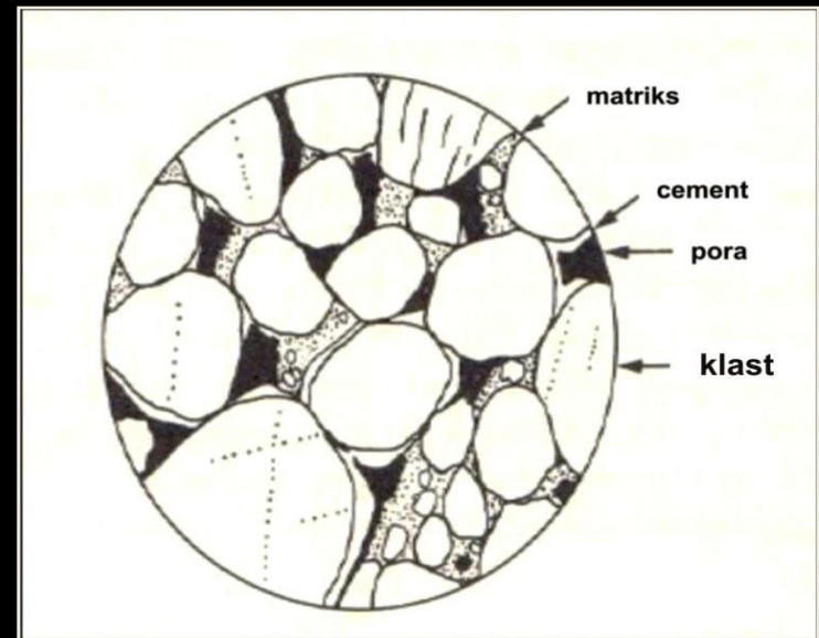
Klastična struktura.
