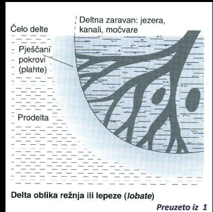
Građa delte.
