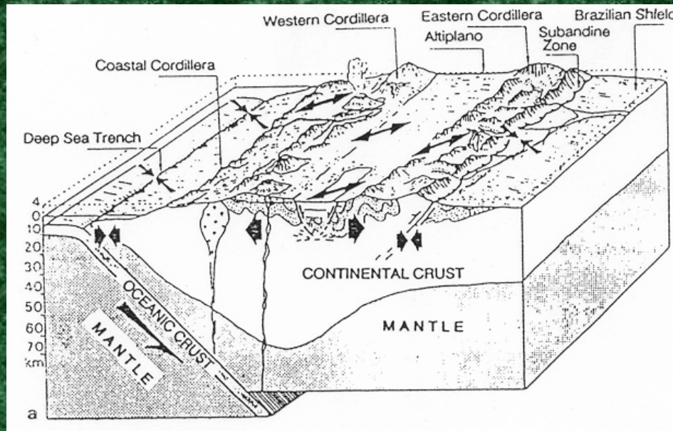
Slika VI-7. Sučeljavanje oceanske i kontinentalne ploče
