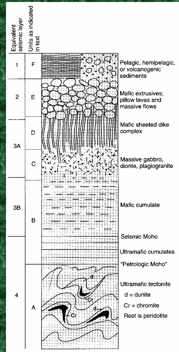
Slika VI-15: Profil kroz ofiolit
