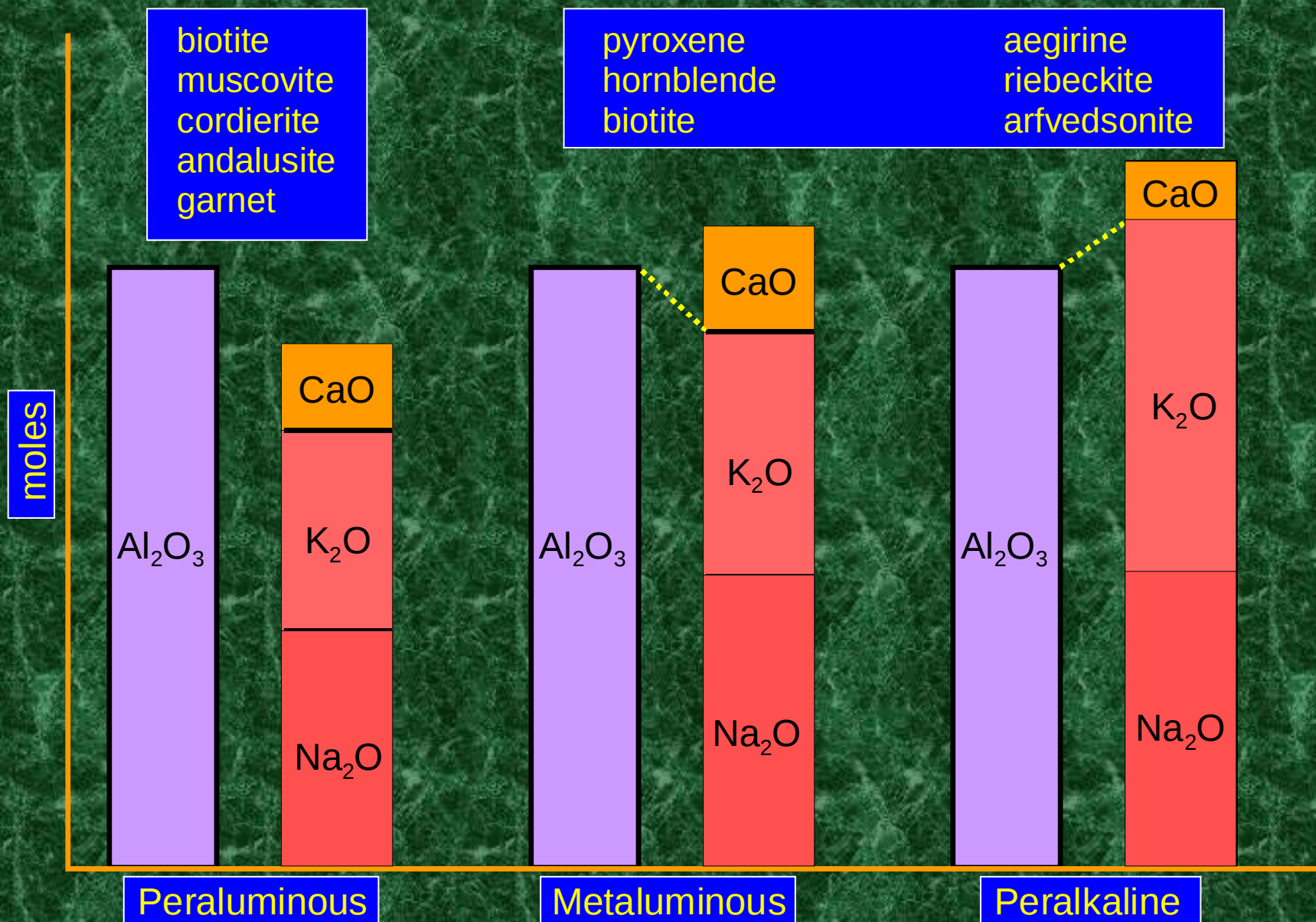
Slika VI-21. Zasićenje aluminijem temelji se na molarnim proporcijama \text{Al}_2\text{O}_3/(\text{CaO}+\text{Na}_2\text{O}+\text{K}_2\text{O}) (“A/CNK”) prema Shand (1927). Za svaki tip su navedeni česti minerali. After Clarke (1992). Granitoid Rocks. Chapman Hall.
