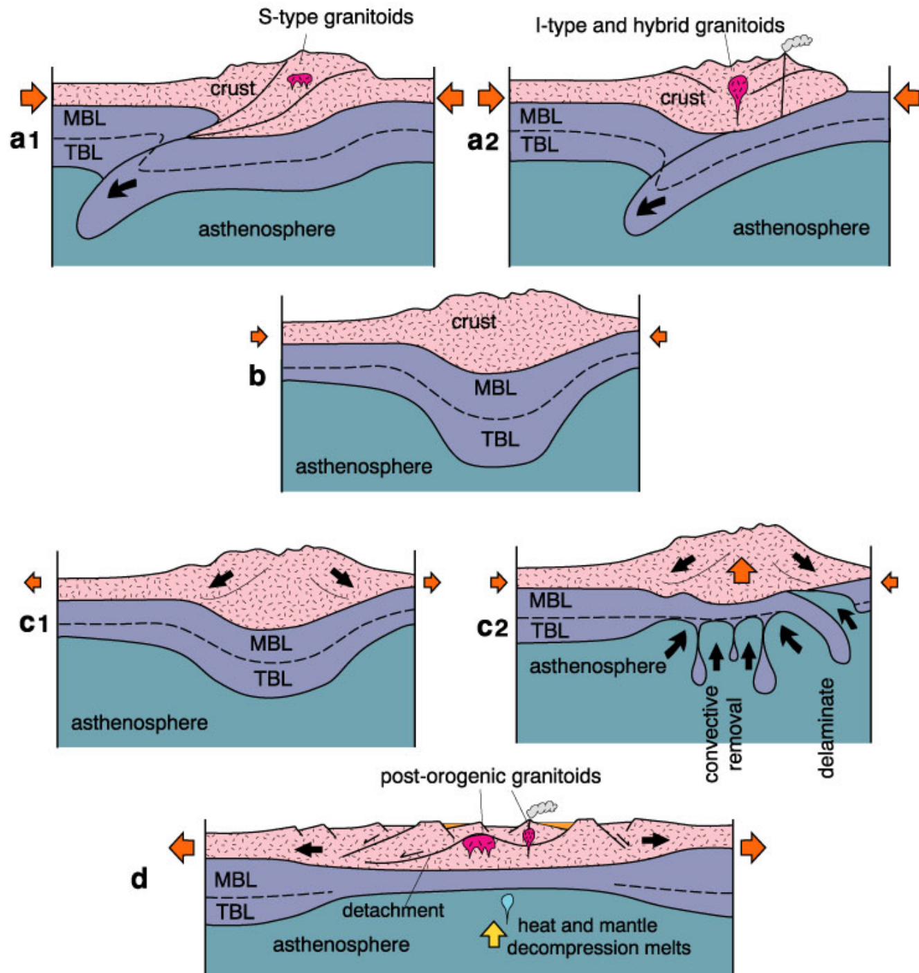
Slika IV-101. Shematski modeli za uzdizanje i ekstenzijski kolaps orogeneze zadebljale kore. Subdukcija vodi do zadebljanja kore kontinentalnom kolizijom (a1) ili kompresijom kontinentalnog luka (a2), svaki od tih modela daje karakterističan orogeni magmatizam. Oba modela vode do zadebljale kore ("MBL" and "TBL" - mechanical and thermal boundary layers) kao u (b). Nakon stabilne situacije u (b), ili se kompresija smanjuje (c1) ili se gusti debeli termalni sloj odstranjuje delaminacijom ili konvektivnom erozijom (c2). Rezultat je ekstenzija i kolaps kore, istanjenje litofsere i uzdizanje vruće astenosfere. (d). Rastući fluks topline (d), plus dekompresijsko taljenje uzdižuće astenosfere rezultira u bimodalnom post-orogenom magmatizmu s bazičnim plašnim magmatizmom i silicijskim magmatizmom iz kore. Winter (2001) An Introduction to Igneous and Metamorphic Petrology. Prentice Hall.
