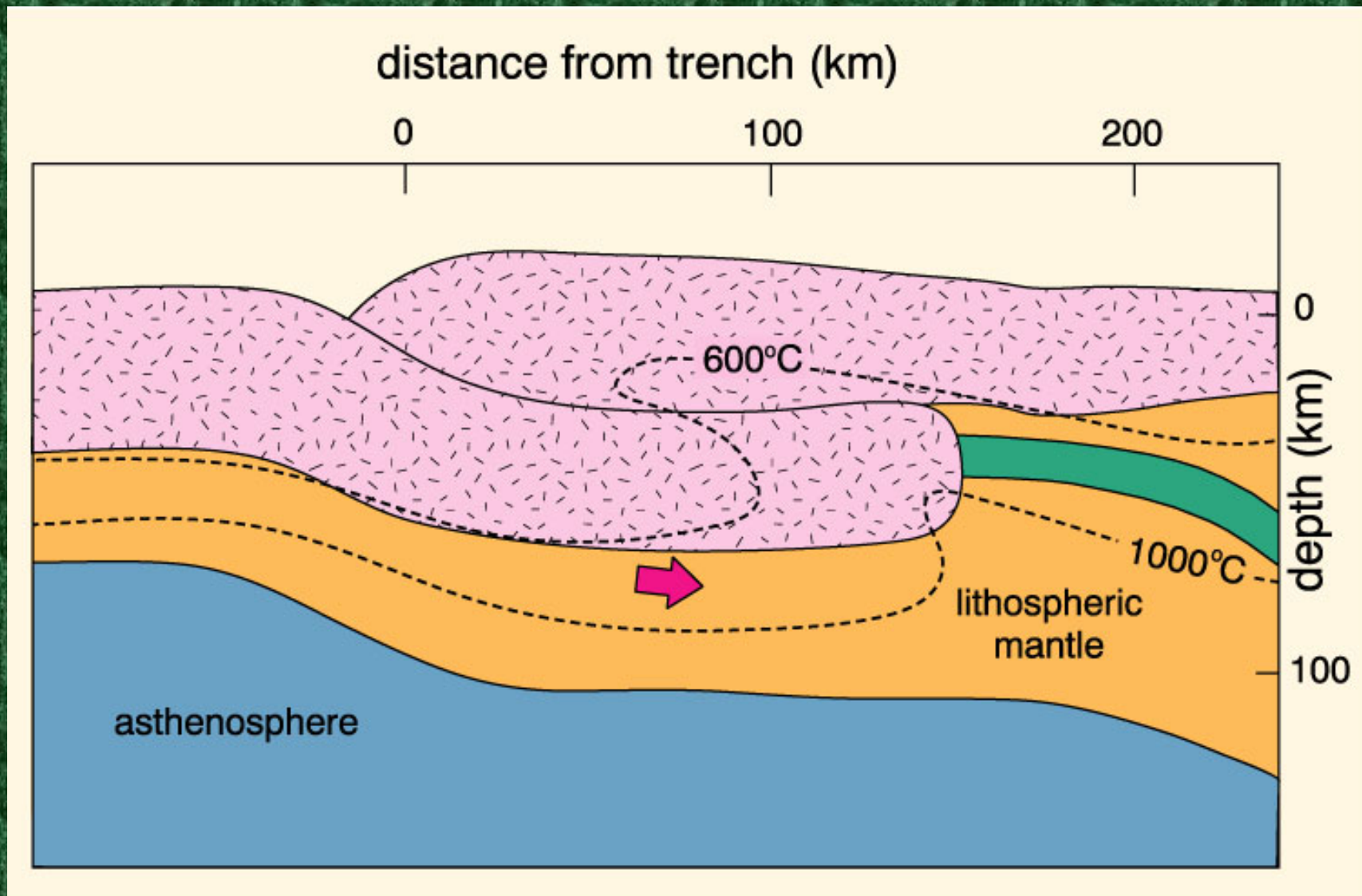
Slika VI-17. Subdukcija kontinentalne kore uzrokuje zadebljanje i dovodi Sial koru na dubinu i temperaturu dovoljnu za uzrokovanje parcijalnog taljenja. Winter (2001) An Introduction to Igneous and Metamorphic Petrology . Prentice Hall.
