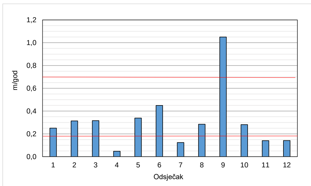
Sl. 4.5. Stope bočnog kretanja odsjeka rijeke u razdoblju 2001. – 2019. Crvene linije predstavljaju prirodne prekide u podacima.
