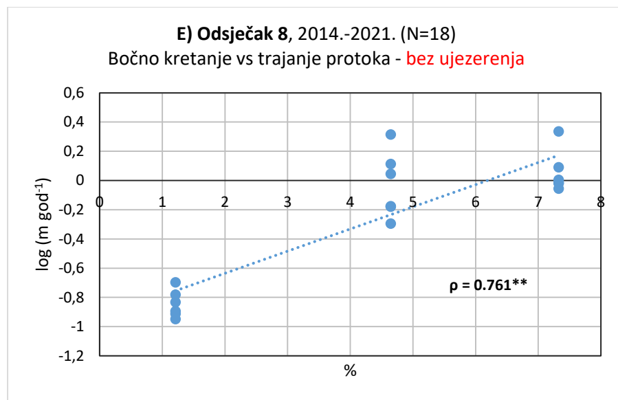
Sl. 4.17. Odnos stope bočnog kretanja i trajanja protoka iznad 25,5 m 3 /s u odsječcima 8 i 9 u istraživanim razdobljima
