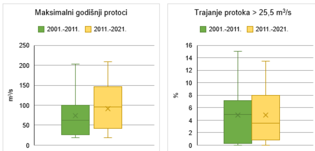
Sl. 4.15. Dijagrami raspona za maksimalne godišnje protoke i trajanje protoka većih od 25,5 \text{ m}^3/\text{s} u razdobljima 2001. – 2011. i 2011. – 2021. na hidrološkoj postaji Frkljevci
