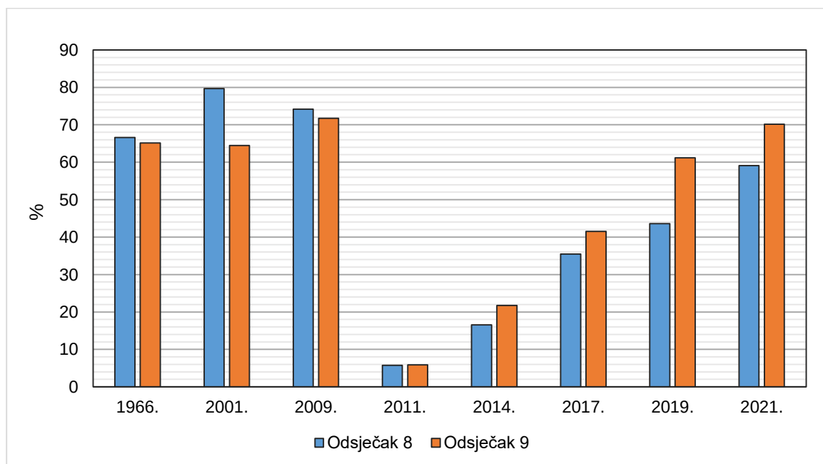
Sl. 4.14. Udjeli drvenaste vegetacije na riječnim obalama u promatranim godinama
