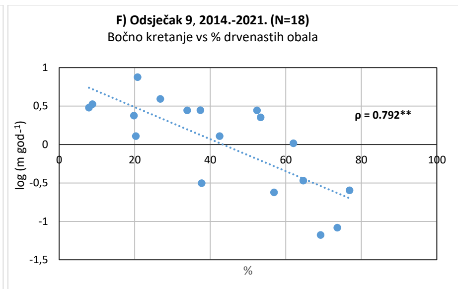
Sl. 4.16. Odnos logaritmirane stope bočnog kretanja i postotnog udjela drvenaste priobalne vegetacije u odsječcima 8 i 9 u istraživanim razdobljima
