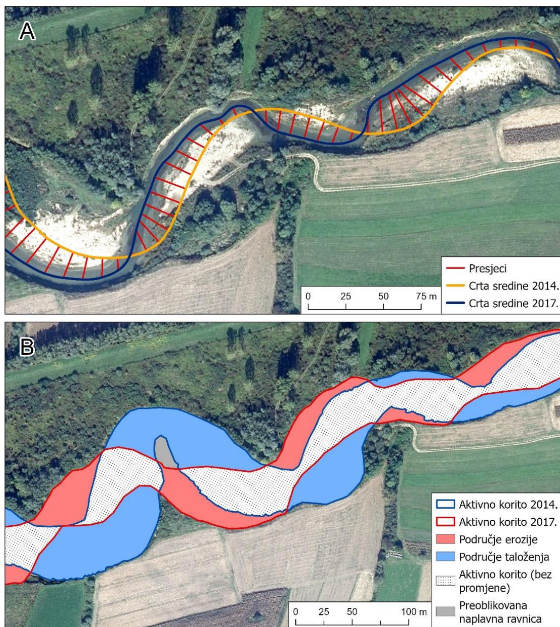
Sl. 3.9. A) Mjerenje lateralnog kretanja rijeke pomoću poprečnih presjeka, B) mjerenje površina erozije i taloženja na temelju preklapanja poligona aktivnog korita iz uzastopnih godina (podloga: ortofoto iz 2017. godine)
