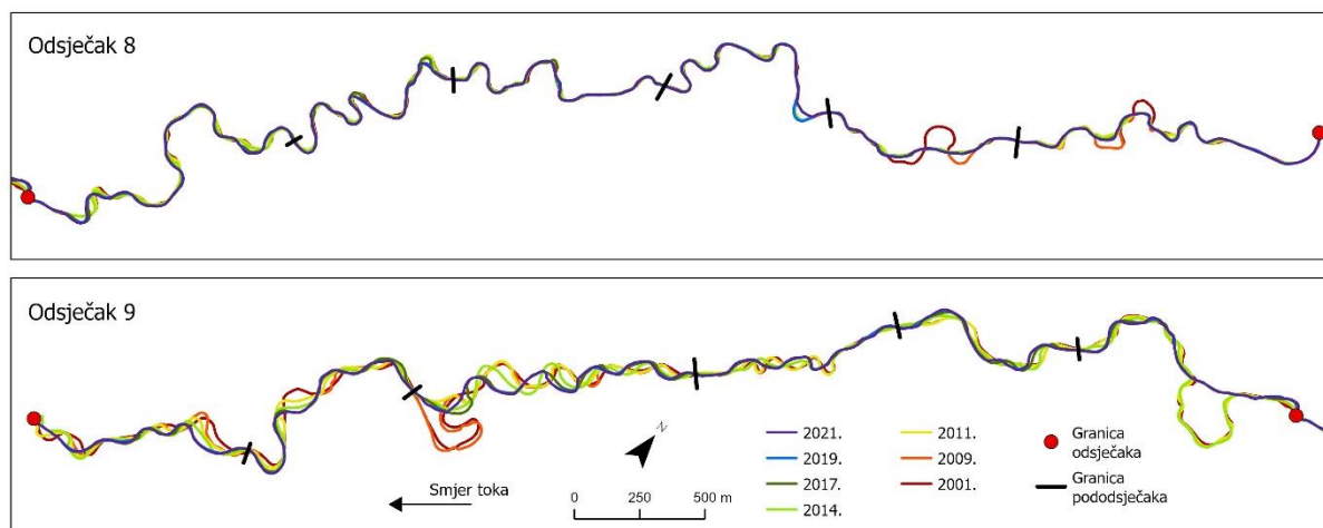
Sl. 3.10. Delineacija pododsječaka unutar odsječaka 8 i 9
