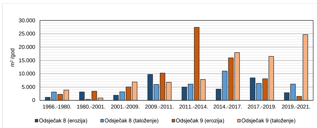
Sl. 4.13. Površine erozije i taloženja u promatranim razdobljima
