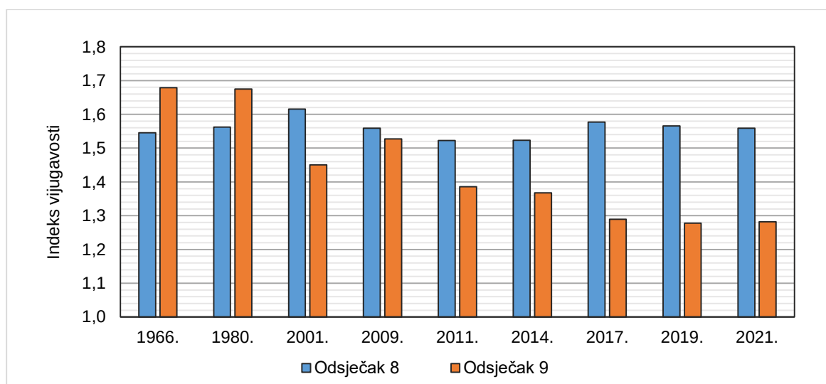
Sl. 4.9. Indeks vijugavosti
