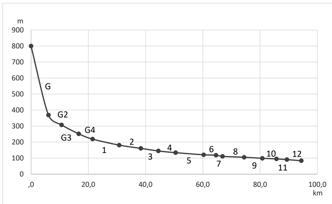
Sl. 3.2. Longitudinalni profil rijeke Orljave od izvora do ušća (na temelju DEM10)
