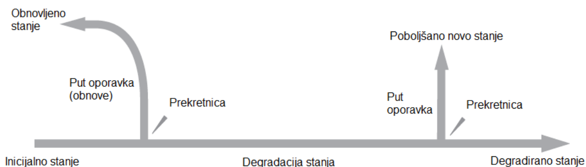
Sl. 5.3. Dijagram potencijala za oporavak rijeke (prema Fryirs i Brierley, 2016)
