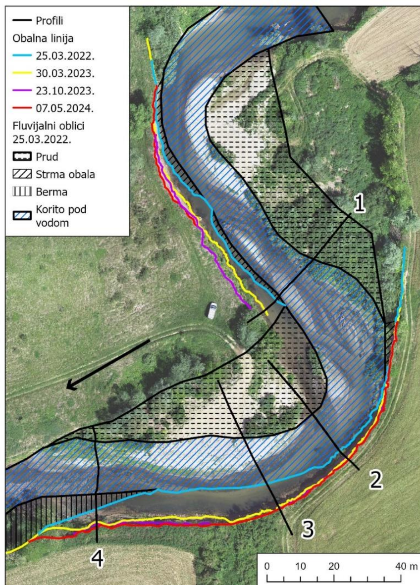
Sl. 4.33. Promjene korita Orljave na lokaciji Bučje, uzvodni meandri, od 2022. do 2024. godine (strelica prikazuje smjer toka). U pozadini ortofoto od 7. 5. 2024.
