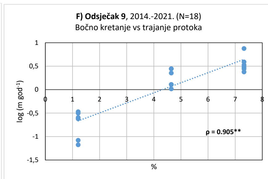
Sl. 4.17. Odnos stope bočnog kretanja i trajanja protoka iznad 25,5 m 3 /s u odsječcima 8 i 9 u istraživanim razdobljima
