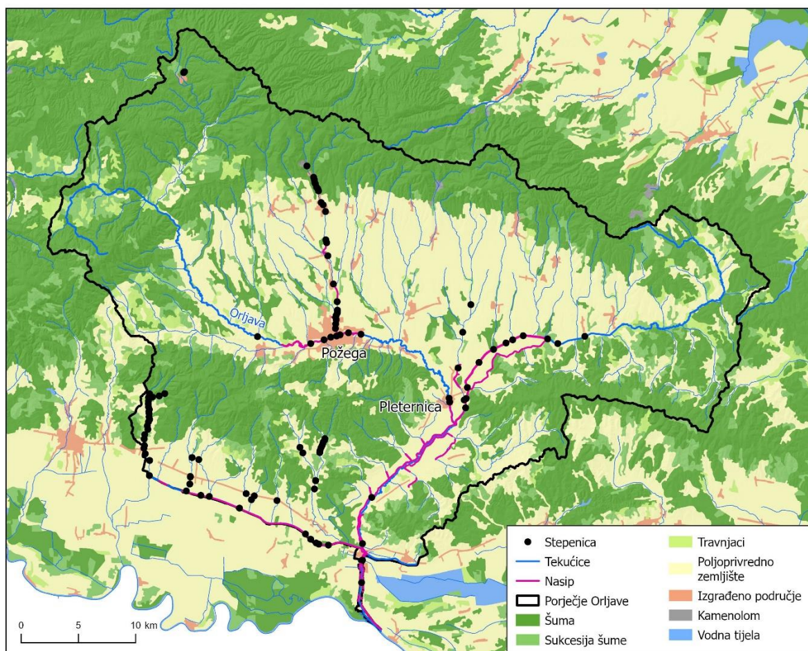
Sl. 2.8. Zemljišni pokrov i hidrotehničke građevine u porječju Orljave. Izvor: Corine Land Cover 2018 (EEA); prostorna baza podataka hidrotehničkih građevina (Hrvatske vode)
