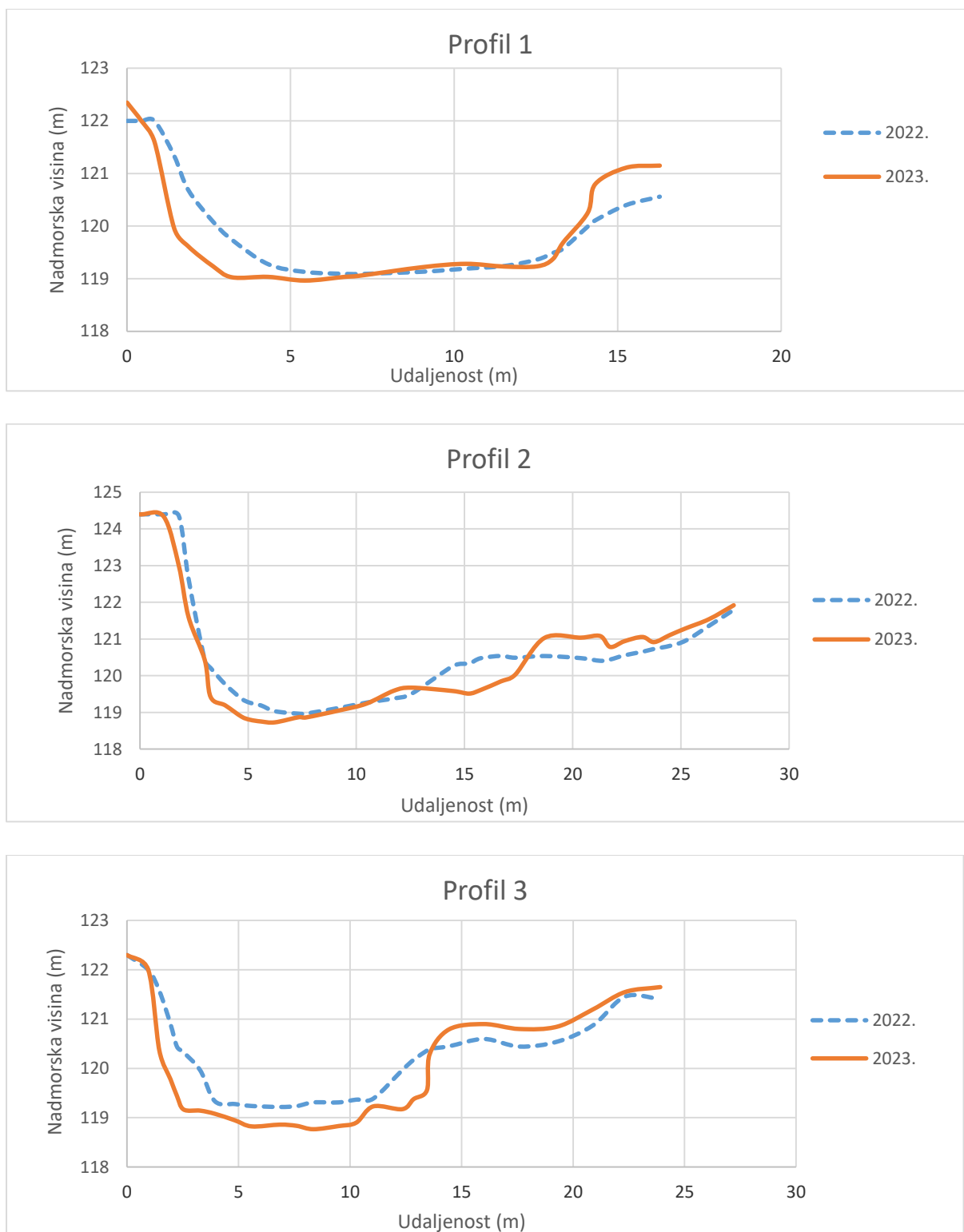
Sl. 4.30. Izmjereni profili na lokaciji Vesela. Isprekidane linije prikazuju profile procijenjene na temelju DSM modela dobivenog snimanjem bespilotnom letjelicom. Svi profili su orijentirani u smjeru toka rijeke (lijeva obala – desna obala).
