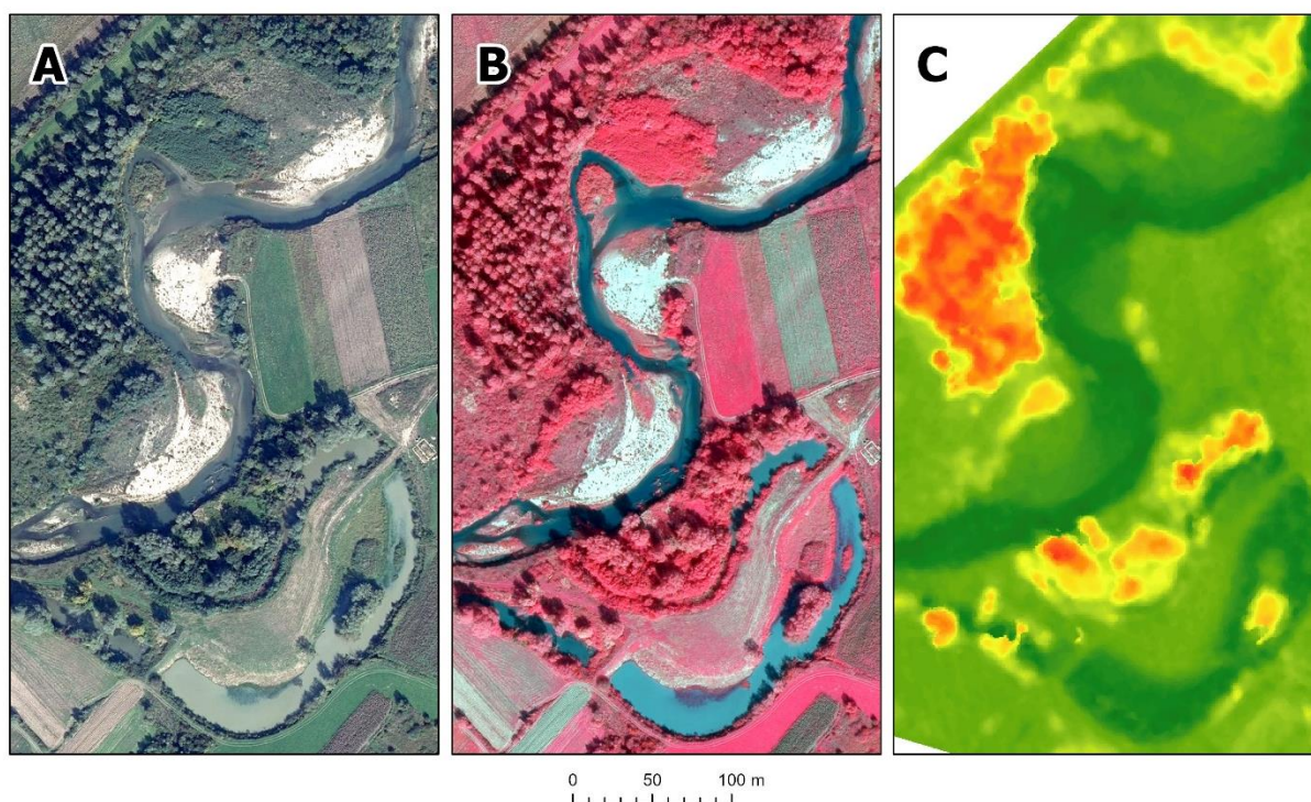
Sl. 3.5. Isječak riječnog koridora Orljave na RGB ortofoto kompozitu za 2017. (A), NIR ortofoto kompozitu za 2017. (B), DDSM-u za 2017. (C)
