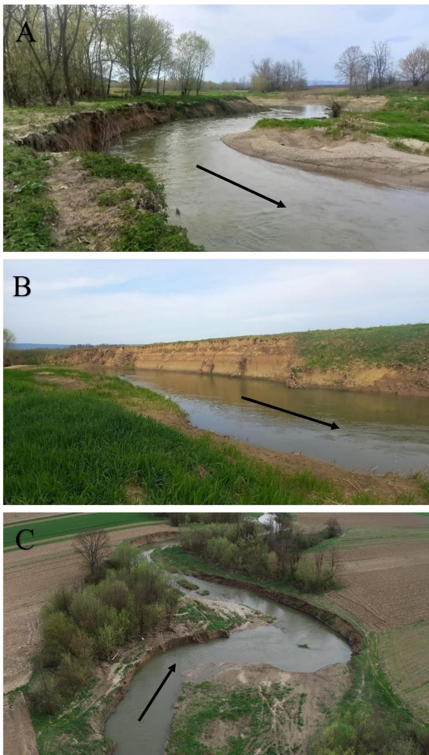
Sl. 4.27. Pogled uzvodno na strmu desnu obalu na uzvodnom dijelu istraživane lokacije (A), strma lijeva obala na središnjem ravnom dijelu istraživane lokacije (B), pogled nizvodno (C). Strelica – smjer toka.
