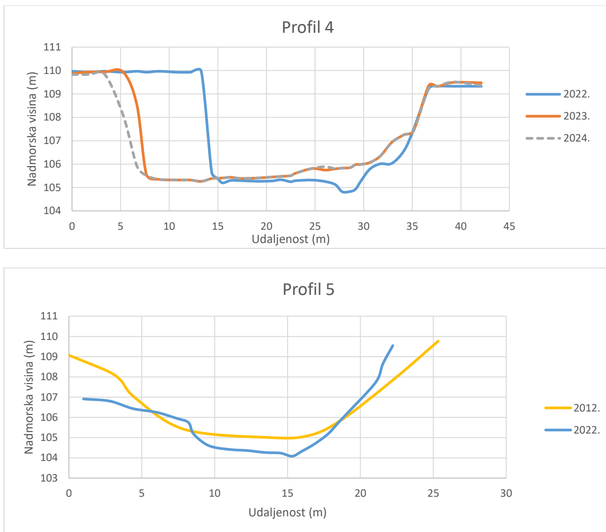
Sl. 4.34. Izmjereni profili na lokaciji Bučje. Isprekidane linije prikazuju profile procijenjene na temelju DSM modela dobivenog snimanjem bespilotnom letjelicom. Svi profili su orijentirani u smjeru toka rijeke (lijeva obala – desna obala).
