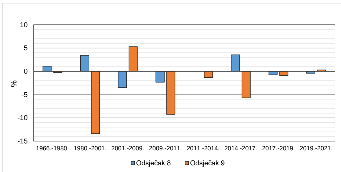
Sl. 4.10. Relativna razlika u duljini korita i indeksu vijugavosti u promatranim razdobljima
