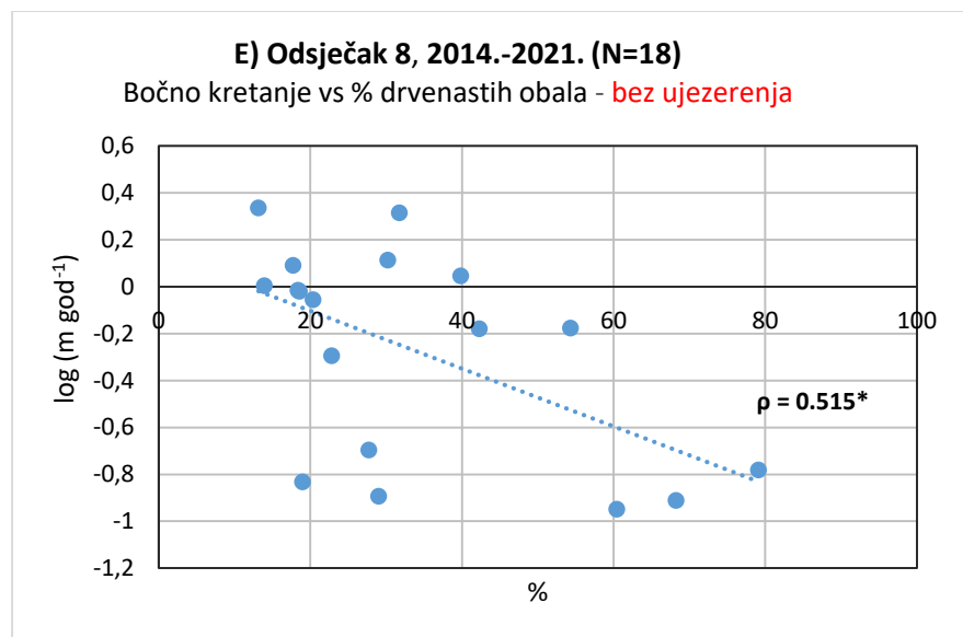
Sl. 4.16. Odnos logaritmirane stope bočnog kretanja i postotnog udjela drvenaste priobalne vegetacije u odsječcima 8 i 9 u istraživanim razdobljima
