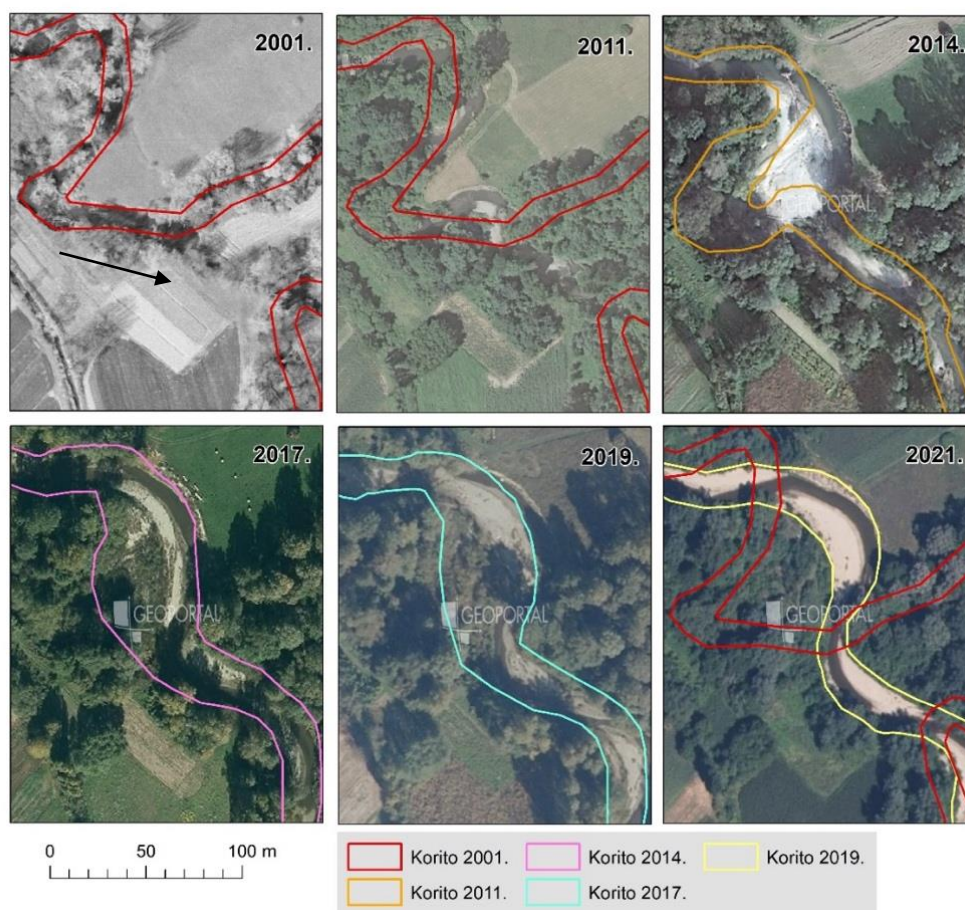
Sl. 4.24. Recentne promjene korita Orljave na lokaciji Boričevci u razdoblju 2001. – 2021.
