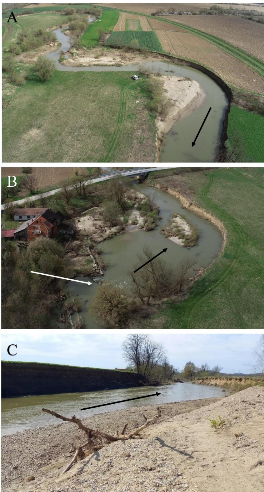
Sl. 4.31. Meandri uzvodno od mlinske stepenice (A), korito nizvodno od stepenice (B), akumulirani sediment i drvni ostaci na prudu (C). Crne strelice označavaju smjer toka, a bijela strelica razrušenu stepenicu. Snimljeno 30. 3. 2023.
