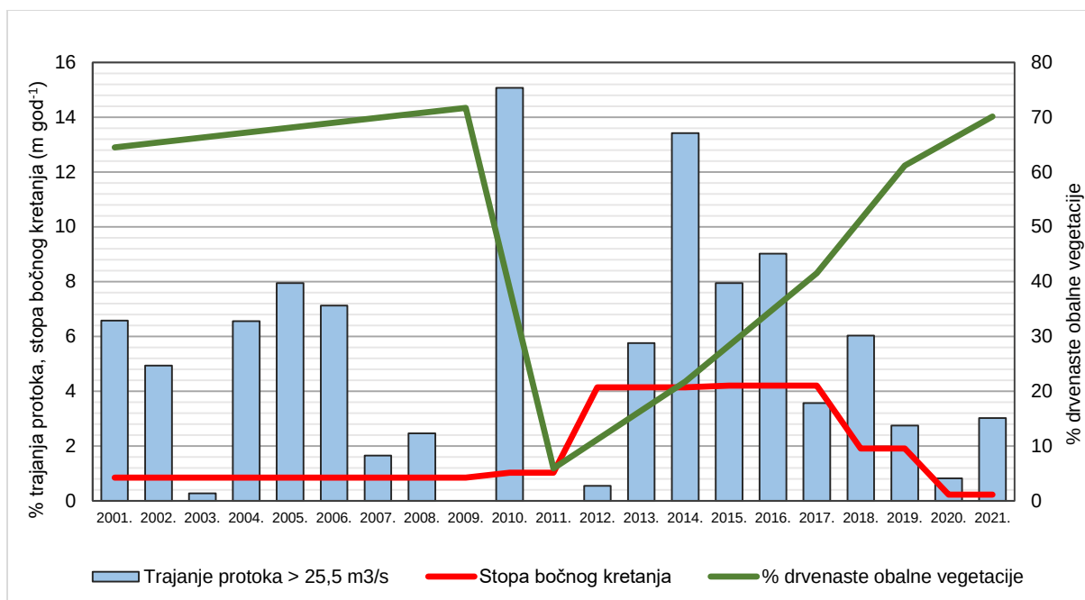
Sl. 5.2. Vrijednosti trajanja protoka iznad 25,5 m 3 /s, stopa bočnog kretanja i udjela drvenaste obalne vegetacije u razdoblju 2001. – 2021. u odsječku 9
