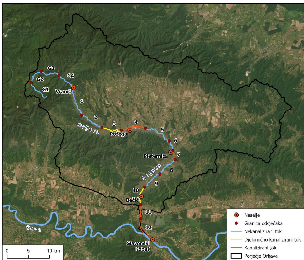
Sl. 3.1. Delineacija odsječaka na toku rijeke Orłjave
