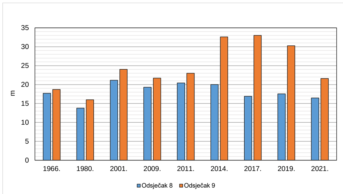
Sl. 4.12. Širina aktivnog korita u promatranim godinama
