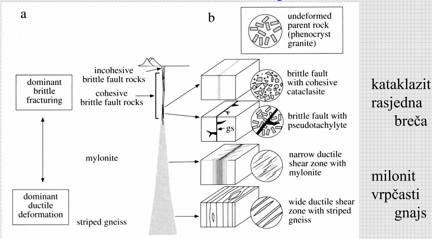
Slika 22-2. Shematski prikaz rasjedne ( shear ) zone pokazuje vertikalnu raspodjelu tipova stijena od nevezanih stijena i breča blizu površine do vezanih i škriljavih stijena. Širina smične zone raste s dubinom te ona postaje elastičnija ( ductile ). U krugovima su prikazane mikrostrukture. Prema Passchier and Trouw (1996) Microtectonics . Springer-Verlag, Berlin.
