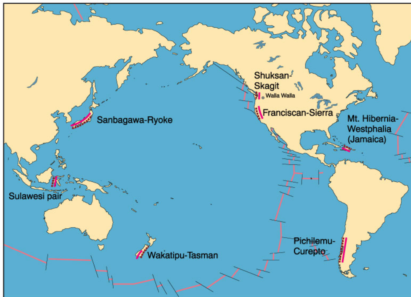
Slika 21-13. Neki od parova metamorfnih pojaseva u circum-Pacifičkom području. Iz Miyashiro (1994) Metamorphic Petrology . Oxford University Press.
