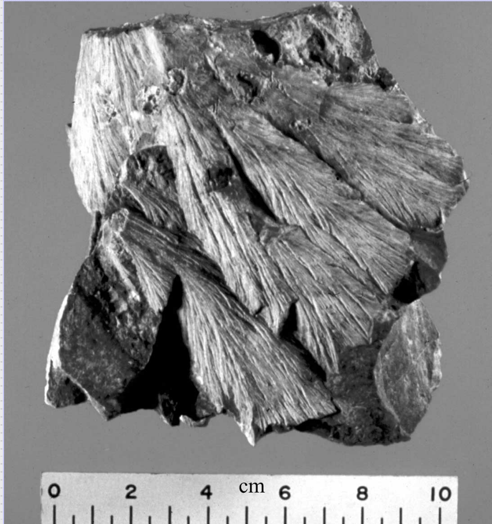
Slika 22-4. Udarni krateri u vapnencu ( shatter cones ) iz Houghton Structure, Northwest Territories. Fotografija: Richard Grieve, © Natural Resources Canada.
