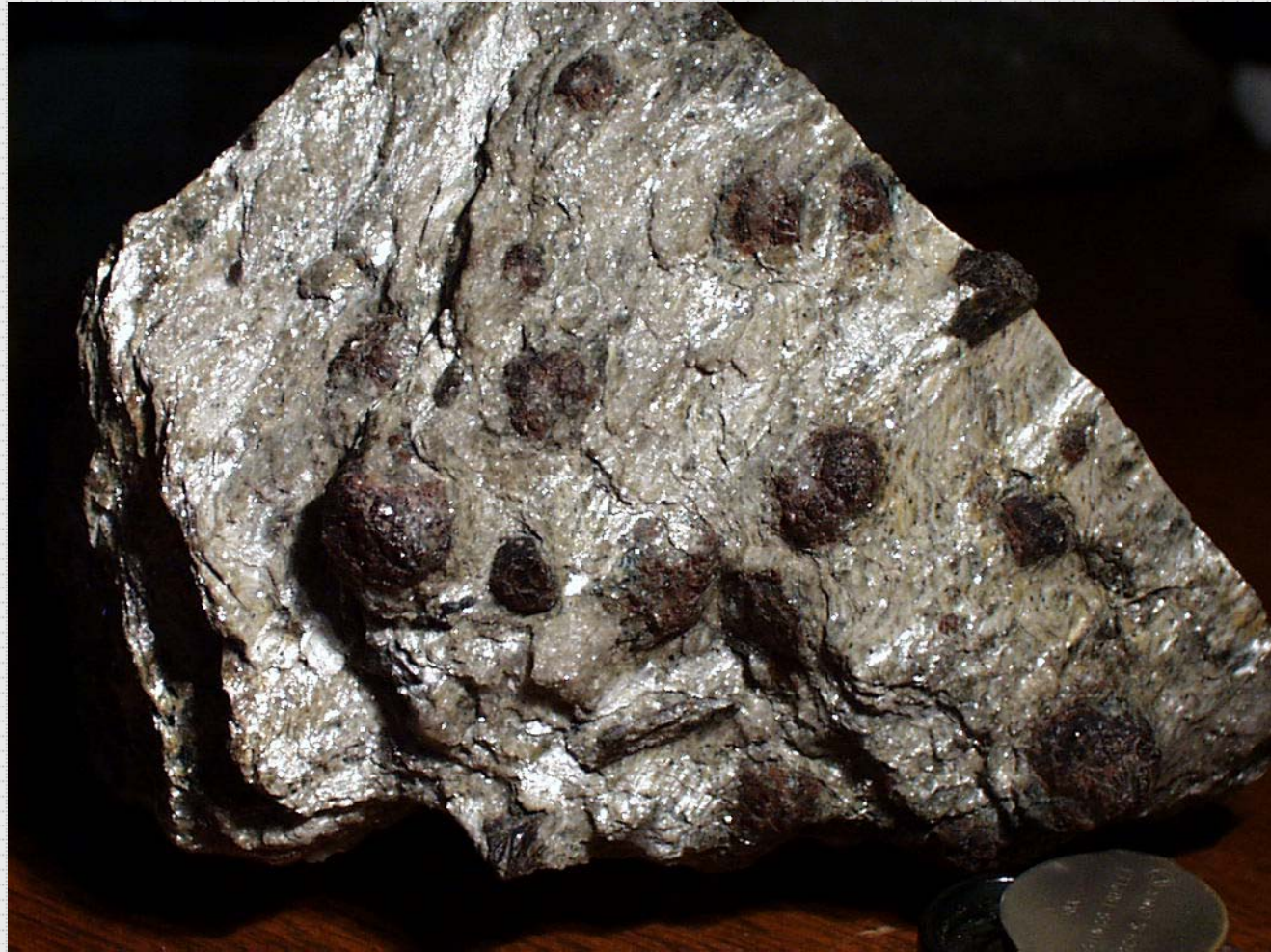
Slika 22-1c. Granat-muskovitski škriljavac. Muskovit daje škriljavost i srebrnkast sjaj stijeni, granati se javljaju kao porfiroblasti. Winter (2001) An Introduction to Igneous and Metamorphic Petrology. Prentice Hall.
