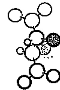
Apsolutna konfiguracija L(+)-tartaratnog iona (1951.)
