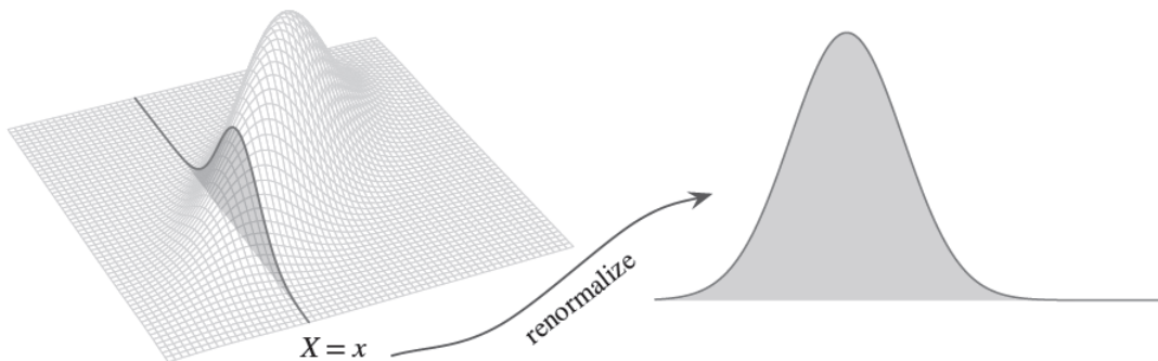
SLIKA 19. Integral osjenčanog dijela (po y ) na lijevoj slici je upravo vrijednost marginalne gustoće f_X(x) iz (8.4). S druge strane, gustoću od Y uz dano X = x dobijemo tako da funkciju y \mapsto f_{X,Y}(x, y) normaliziramo tako da postane dobro definirana gustoća. Preuzeto iz [BH19].
