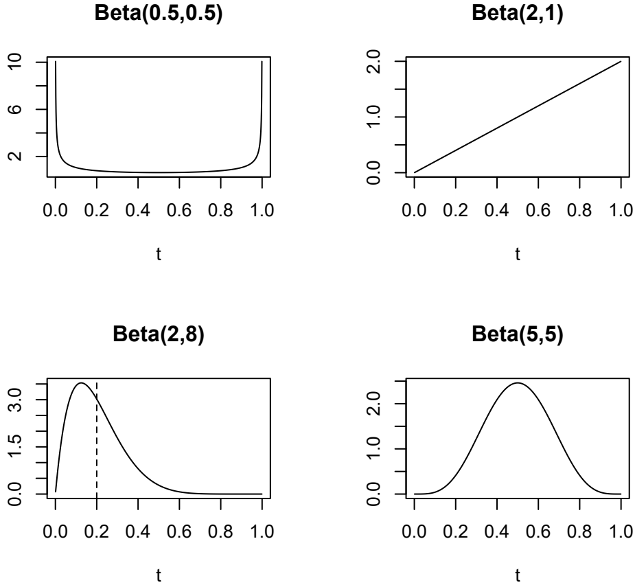
SLIKA 20. Gustoća \text{Beta}(a, b) za nekoliko kombinacija parametara a, b > 0 . U slučaju a = 2, b = 8 , vertikalnom linijom je naznačeno očekivanje a/(a+b) = 0.2 .
