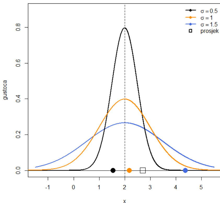
SLIKA 8. Na slici je nacrtano n = 3 normalnih gustoća s istim očekivanjem \mu = 2 te različitim varijancama, a na x -osi su po jedna realizacija slučajne varijable iz svake od te tri distribucije. Cilj je iz tih realizacija što bolje odrediti \mu (koji ne znamo unaprijed).
