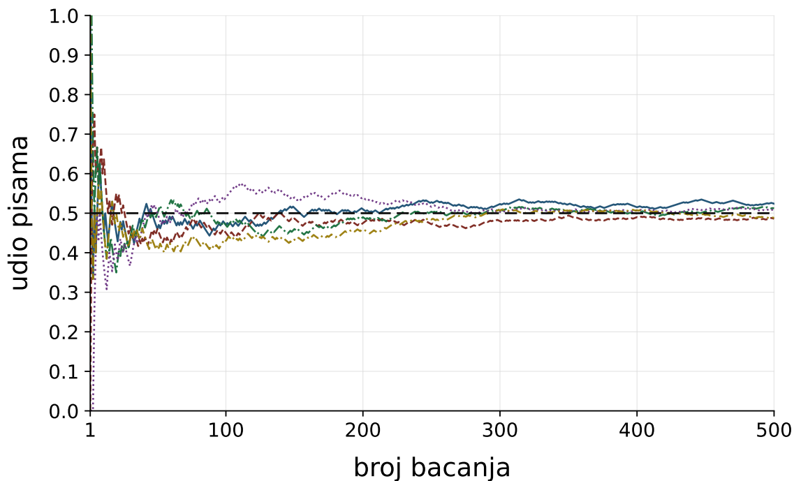
SLIKA 9. Simulirali smo 5 nizova bacanja simetričnog novčića (dakle, p = 0.5 ) te smo prikazali udio pisama \bar{X}_n u ovisnosti o broju bacanja n za n = 1, 2, \dots, 500 .
