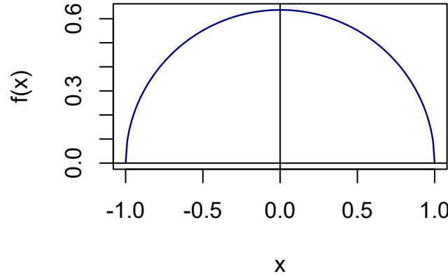
SLIKA 18. Gustoća f(x) = \frac{2}{\pi} \sqrt{1-x^2} za x \in [-1, 1] .
