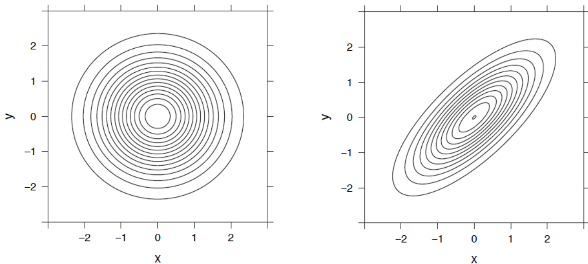
SLIKA 23. Alternativan prikaz gustoća sa Slike 22 koristeći konture konstantne gustoće. Ako je f : \mathbb{R}^2 \rightarrow [0, \infty) gustoća, gornje linije ( konture ) su skupovi \{(x, y) : f(x, y) = c\} za nekoliko različitih izbora konstante c > 0 . Drugim riječima, konture dobijemo tako da graf funkcije f presječemo s ravninom z = c . Konture gustoće standardne dvodimenzionalne normalne razdiobe (lijevo) su kružnice oko ishodišta jer f(x, y) ovisi samo o normi \|(x, y)\| (tj. udaljenosti od ishodišta). Općenito, konture konstantne gustoće su rotirane elipse (vidi desno). Preuzeto iz [BH19].
