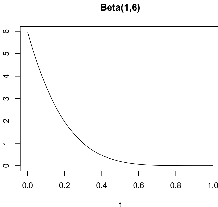
SLIKA 21. Aposteriorna razdioba za P u Primjeru 8.17, i to u slučaju uniformne apriorne razdiobe, n = 5 i N_n = 0 . Dakle, u Bayesovskom pristupu dobivamo cijelu razdiobu za parametra koji procjenjujemo!
