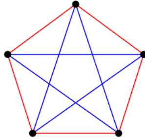
SLIKA 1. Primjer bojanja peterokuta (dakle n = 5 ) za koji ne postoji monokromatski podgraf veličine k = 3 (tj. monokromatski trokut). Dakle, R(3, 3) \geq 5 + 1 = 6 , te je zapravo poznato da vrijedi R(3, 3) = 6 .
