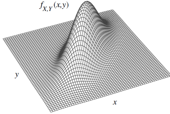
SLIKA 17. Primjer zajedničke gustoće – za svaki A \subseteq \mathbb{R}^2 , \mathbb{P}((X,Y) \in A) je volumen skupa \{(x,y,z) \in \mathbb{R}^3 : (x,y) \in A, 0 \leq z \leq f(x,y)\} . Preuzeto iz [BH19].
